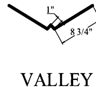
ORV1 20 1/2"
