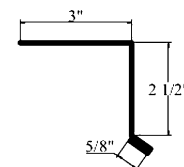
DRIP EDGE
